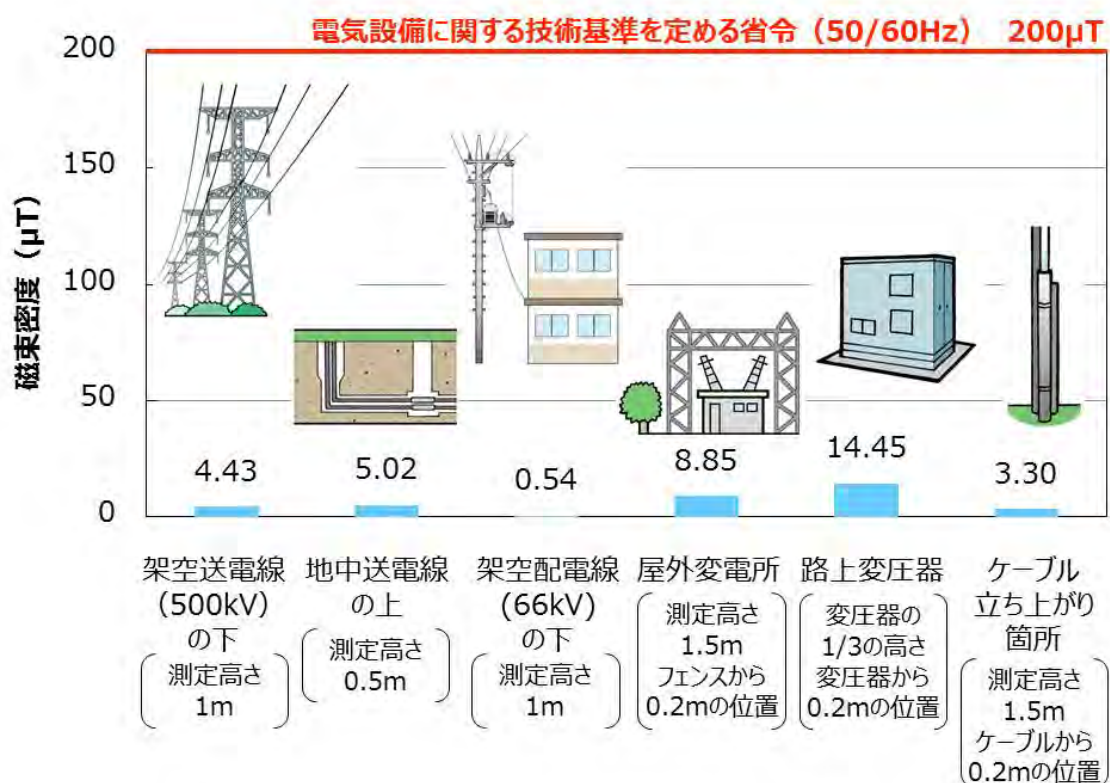
図 4 電力設備からの磁界の強さ(最大値の例)
